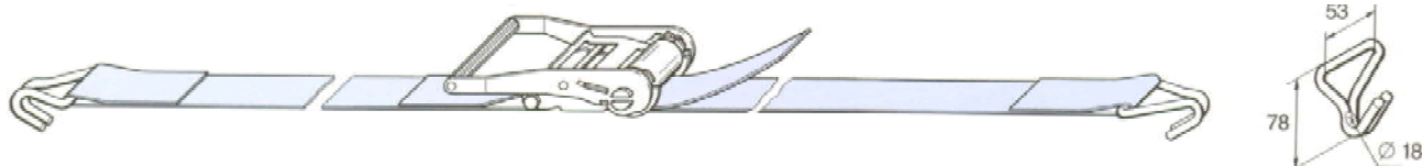
Sangle à tendeur à blocage avec crochets en tréfilé Ratschenschlossgurt mit geschlossenem drahthaken
