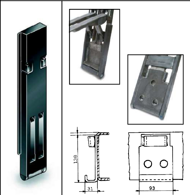
Montanti rovesciabili con battuta di 33 mm per sponde in alluminio Overturing steel pillars of 33 mm for aluminium sideboards Stahl runge in klappbarer Ausführung mit Abschluss 33 mm für All. Bordwände
