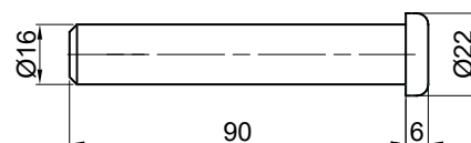
Perno grezzo Ø16 senza foro Raw pin Ø16 without hole
