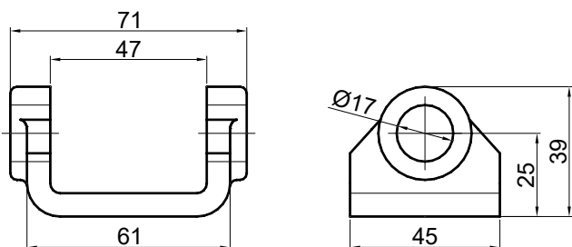
Orecchietta pesante grezza Raw heavy ear
