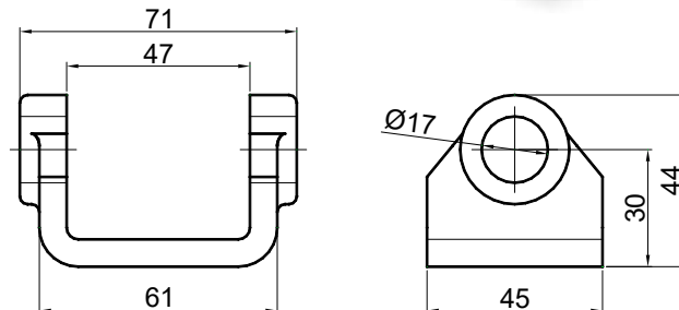
Saltarello ferma leva grezzo Raw click
