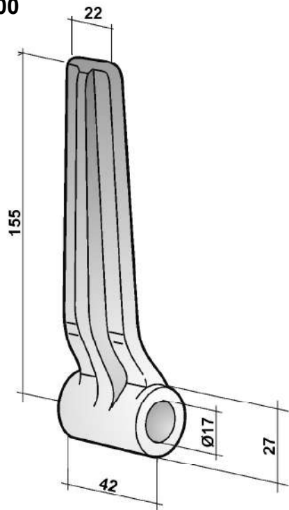
Cerniera grezza tipo Salerno Ø 17 Raw Salerno hinge Ø 17
