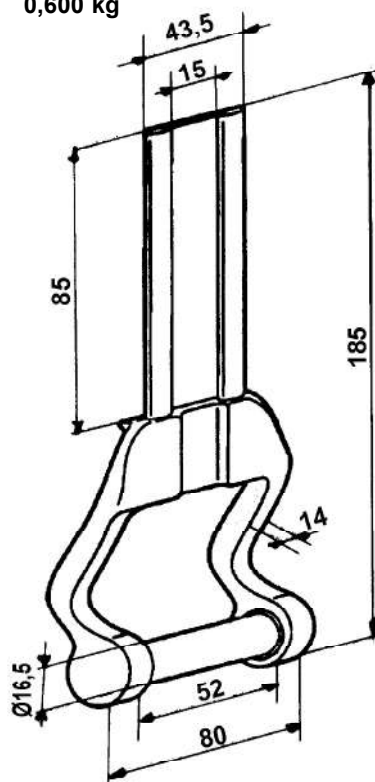
Cerniera grezza Raw hinge
